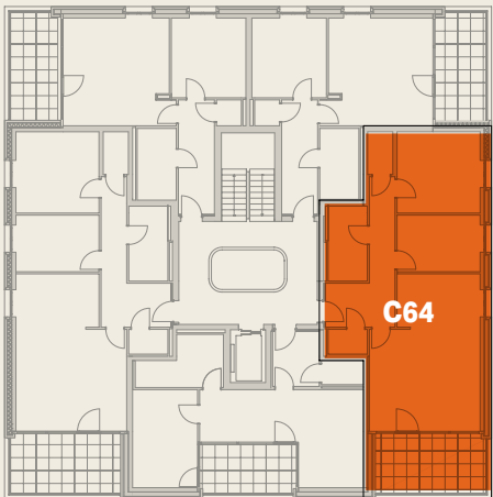
Geschossplan 2.OG
