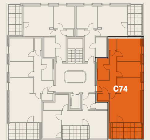
Geschossplan 4.OG
